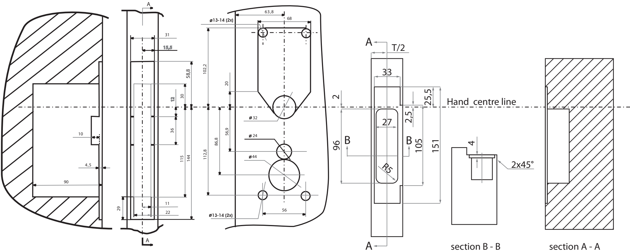
SEKCIJA A-A
